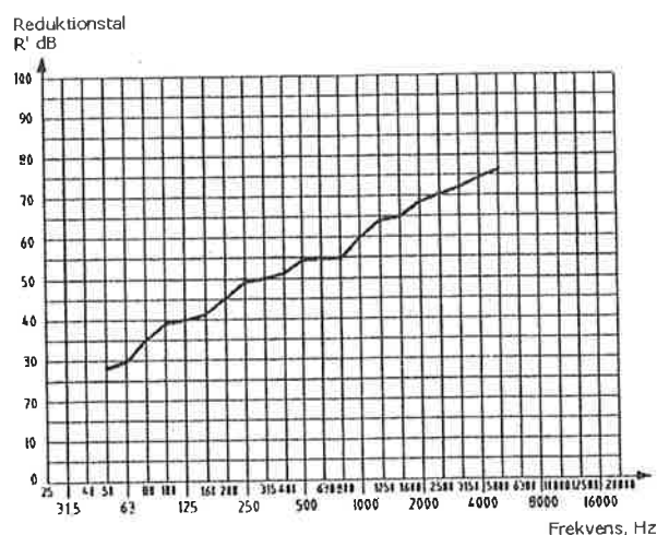
Figur 2. Typisk reduktionstalskurva för skiljekonstruktion utan läckor.
