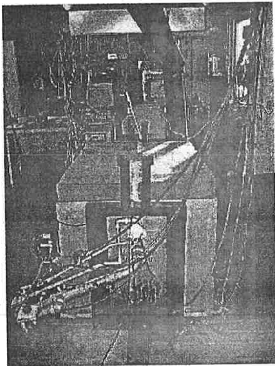
Figur 11. Träteks laboratorieugn för brandprov
