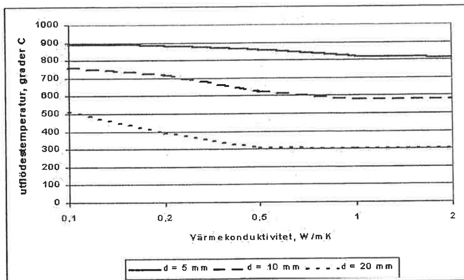
Figur 9. Utflödestemperaturen som funktion av värmekonduktiviteten för väggmaterialet, för tre olika håldiametrar.
