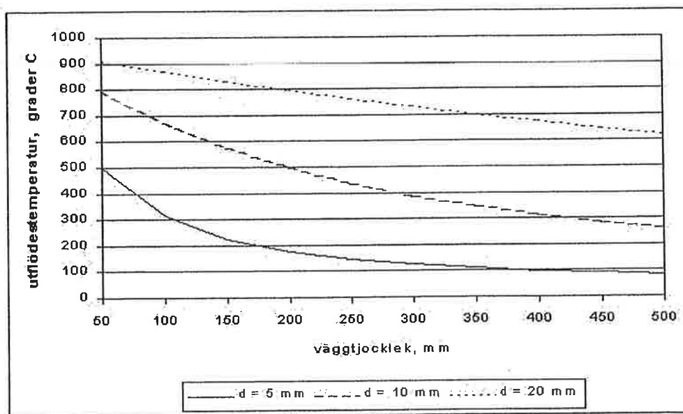
Figur 8. Utflödestemperaturen som funktion av vägg tjockleken, för tre olika håldiametrar.
