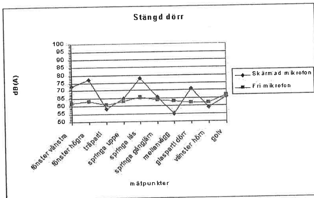
Figur 4. Jämförelse mellan mätningar med skärmad och med fri mikrofon på väggen i figur 3.
