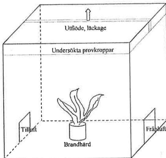
Figur 10. Principmodell över brandugn
