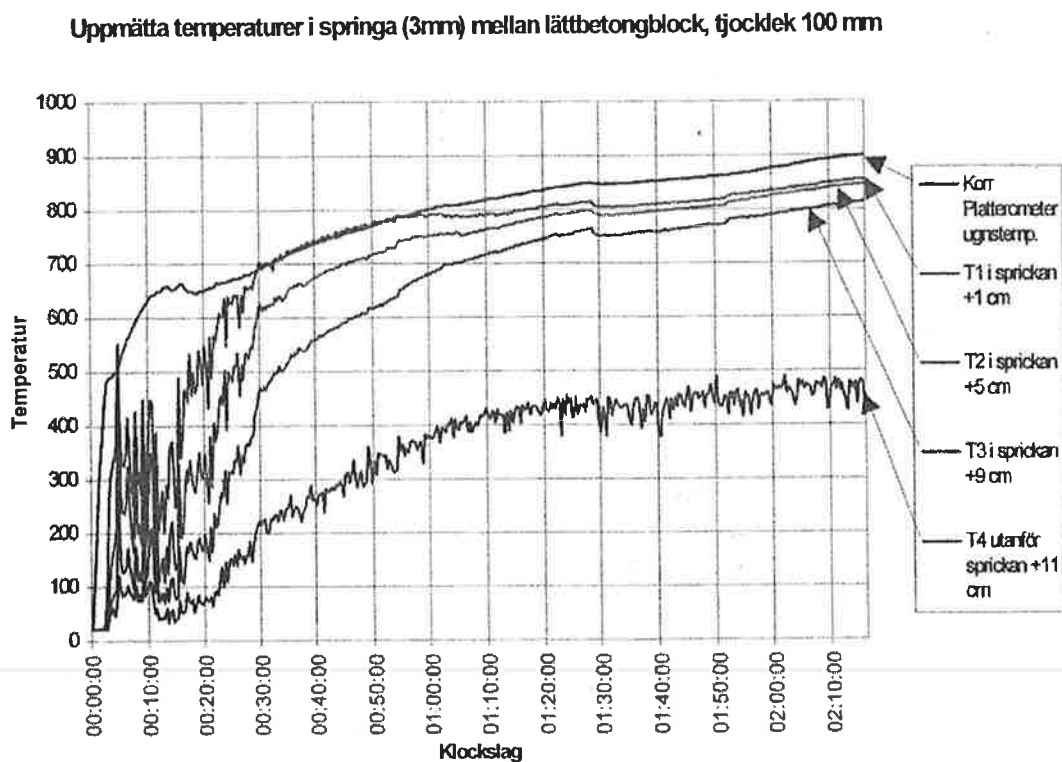
Figur 16. Resultat från prov på lättbetong
