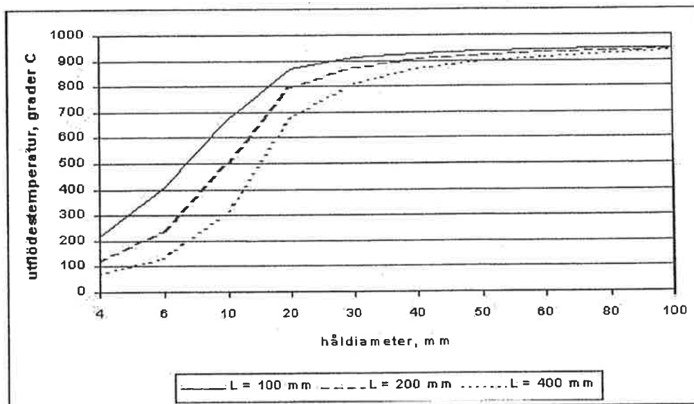
Figur 7. Brandgasens utflödestemperatur som funktion av håldiametern, för tre olika vägg tjocklekar.
