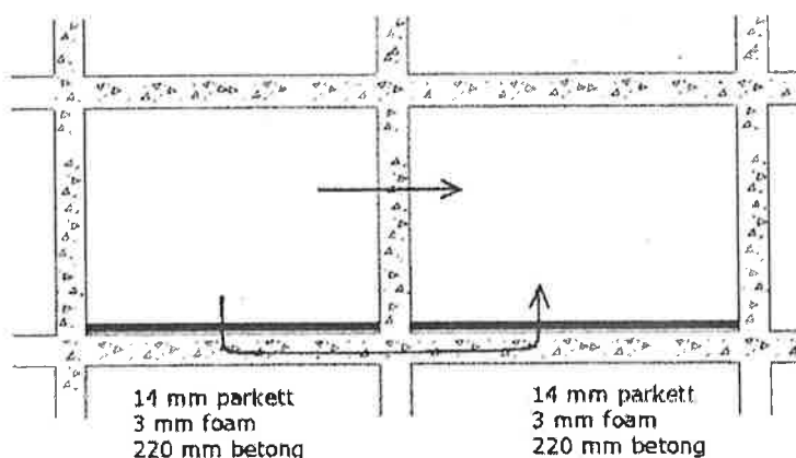
Figur 2. Försämring av ljudisoleringen för en skiljevägg p.g.a. parkettresonans.
