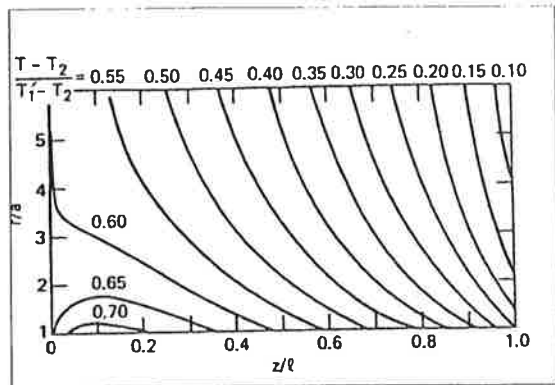
Figur 3 Temperatur konturer i väggen.
